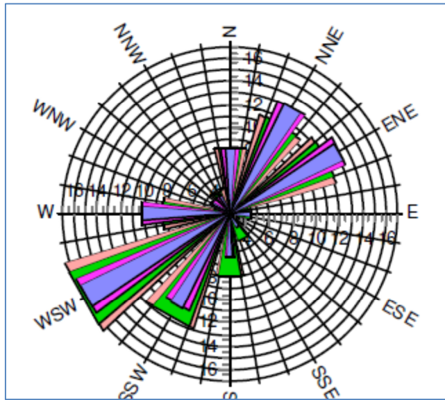
Figure 3 : Distribution des vitesses du vent (Mât de mesures de Fomperron, RP GLOBAL)
